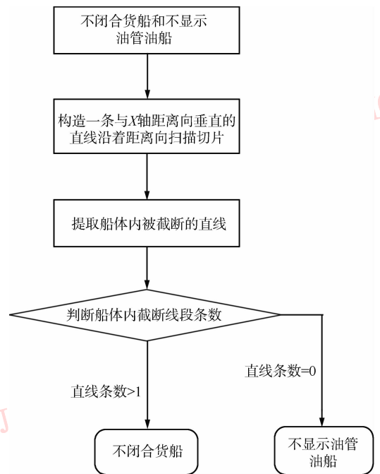
图 5 不显示油管油船和不闭合货船识别流程
