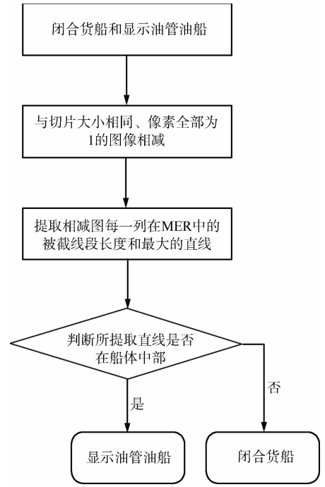
图 4 显示油管油船和闭合货船识别流程
