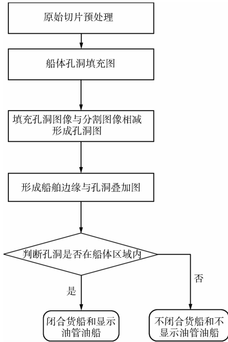
图 2 船舶识别第 1 阶段流程图
